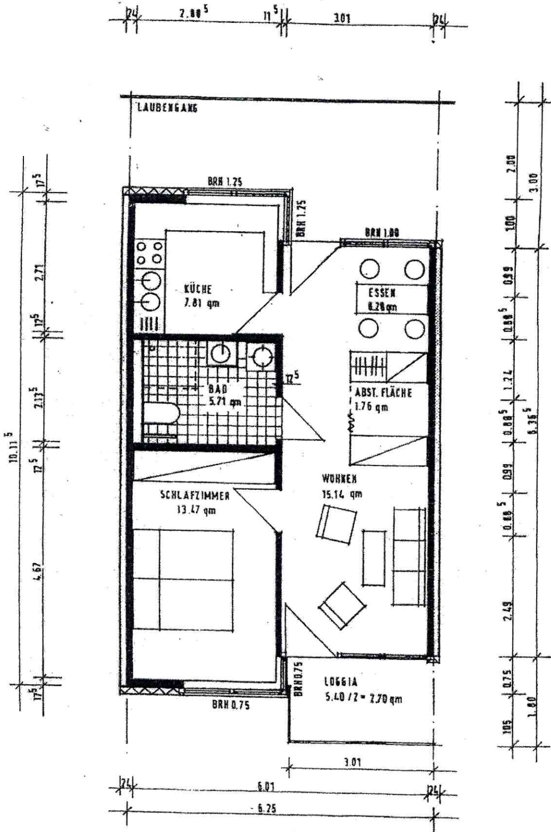
GRUNDRISS 2-ZIMMER-WOHNUNG 54,87 m²
